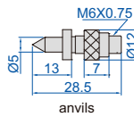
anvils
